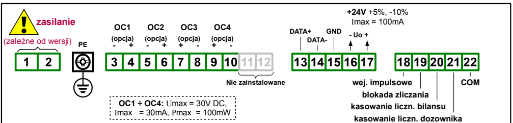
Rys. 4.10. Opis wyprowadzeń dla wersji z czterema wyjściami typu OC
