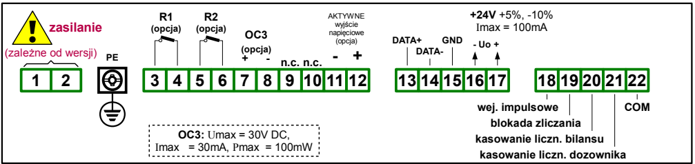
Rys. 4.8. Opis wyprowadzeń dla wersji z dwoma wyjściami przełącznikowymi, wyjściem typu OC oraz aktywnym wyjściem napięciowym
