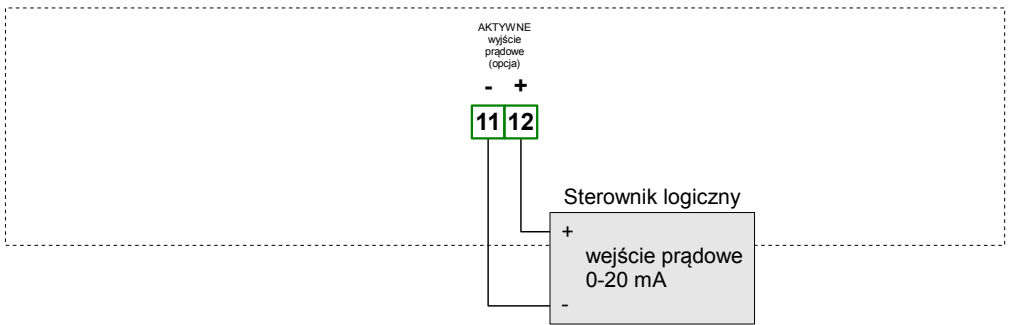
Rys. 4.17. Przykład podłączenia aktywnego wyjścia prądowego (tylko dla urządzeń posiadających aktywne wyjście prądowe)
