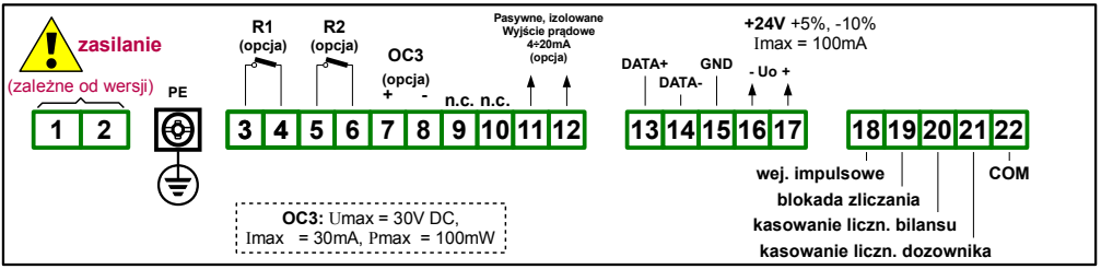
Rys. 4.7. Opis wyprowadzeń dla wersji z dwoma wyjściami przełącznikowymi, wyjściem typu OC oraz pasywnym wyjściem prądowym
