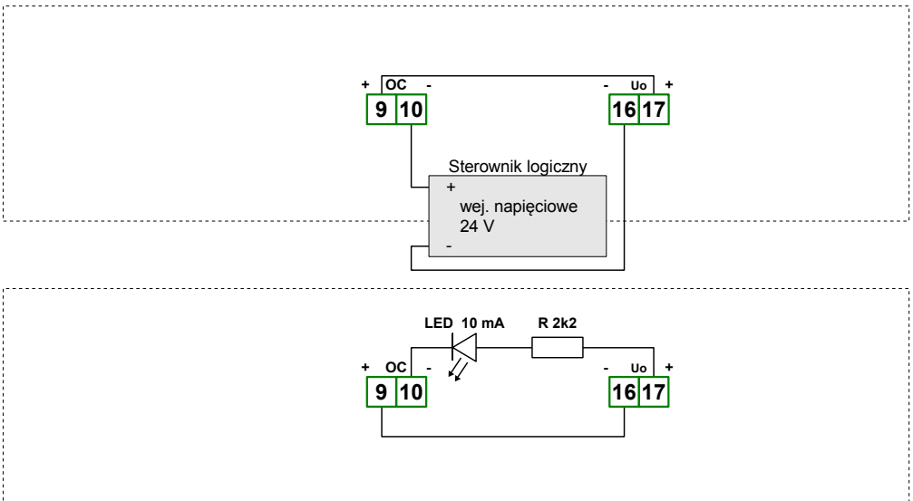
Rys. 4.16. Przykładowe podłączenia wyjścia typu OC (tylko dla urządzeń posiadających wyjście typu OC)
