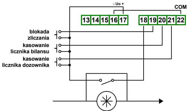
Rys. 4.13. Przykładowe podłączenie przetwornika przepływu z wyjściem kontaktronowym
