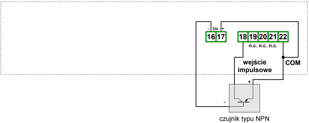
Rys. 4.15. Przykładowe połączenia czujnika ze wspólnym plusem
