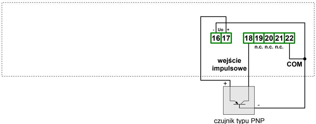
Rys. 4.14. Przykładowe połączenia czujnika ze wspólną masą
