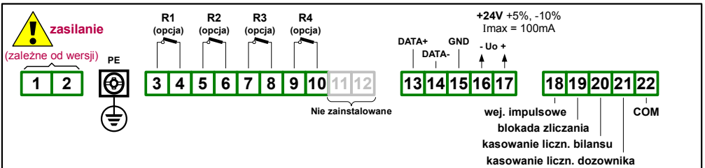
Rys. 4.9. Opis wyprowadzeń dla wersji z czterema wyjściami przełącznikowymi
