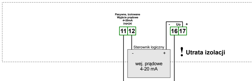
Rys. 4.15. Przykład podłączenia pasywnego wyjścia prądowego (tylko dla urządzeń posiadających pasywne wyjście prądowe)
