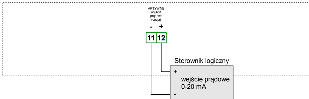
Rys. 4.14. Przykład podłączenia aktywnego wyjścia prądowego (tylko dla urządzeń posiadających aktywne wyjście prądowe)
