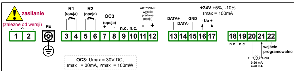
Rys. 4.6. Opis wyprowadzeń dla wersji z dwoma wyjściami przekąźnikowymi, wyjściem typu OC oraz aktywnym wyjściem prądowym
