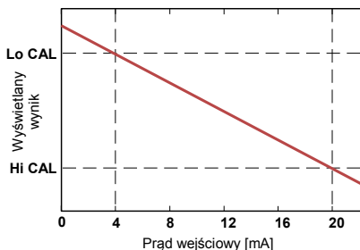
Rys. 9.1 Charakterystyka prosta („Lo CAL” < „Hi CAL”) i odwrócona („Lo CAL” > „Hi CAL”)
