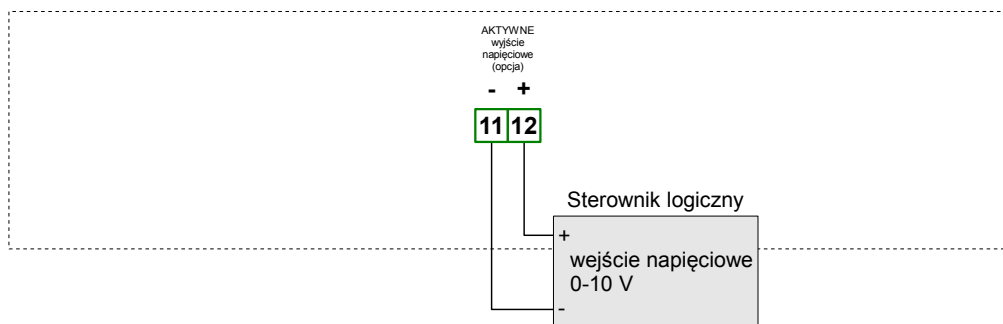
Rys. 4.16. Przykład podłączenia aktywnego wyjścia napięciowego (tylko dla urządzeń posiadających aktywne wyjście napięciowe)
