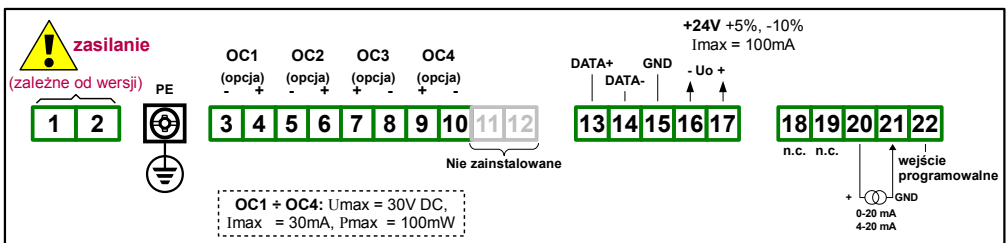
Rys. 4.10. Opis wyprowadzeń dla wersji z czterema wyjściami typu OC
