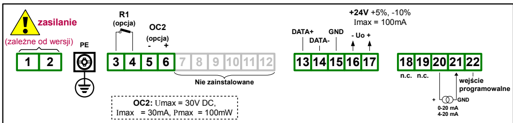
Rys. 4.5. Opis wyprowadzeń dla wersji z wyjściem przekąźnikowym i wyjściem typu OC
