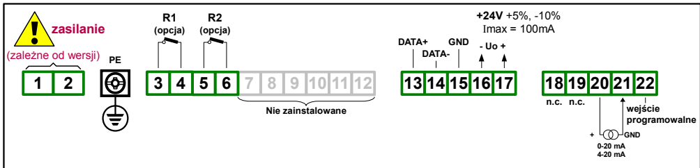
Rys. 4.3. Opis wyprowadzeń dla wersji z dwoma wyjściami przekąźnikowymi
