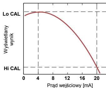
Rys. 9.2 Charakterystyka prosta („Lo C” < „Hi CAL”) i odwrócona („Lo C” > „Hi CAL”)
