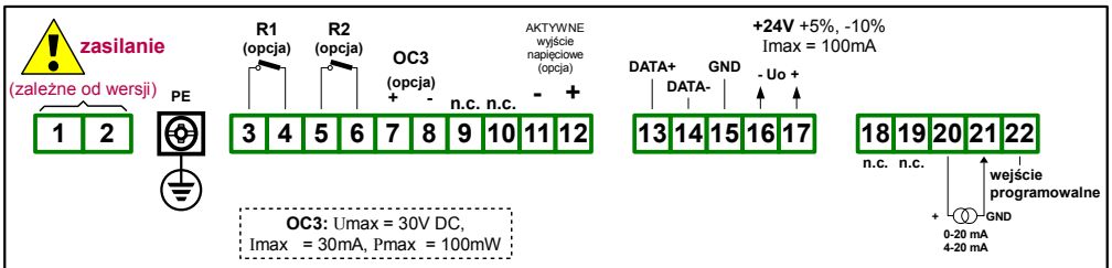
Rys. 4.8. Opis wyprowadzeń dla wersji z dwoma wyjściami przełącznikowymi, wyjściem typu OC oraz aktywnym wyjściem napięciowym
