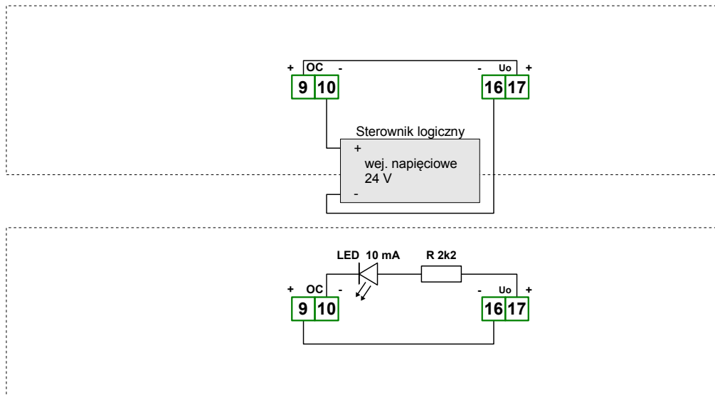
Rys. 4.13. Przykładowe podłączenia wyjścia typu OC (tylko dla urządzeń posiadających wyjście typu OC)
