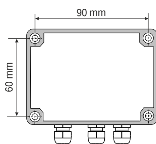
Rozstaw otworów mocujących
